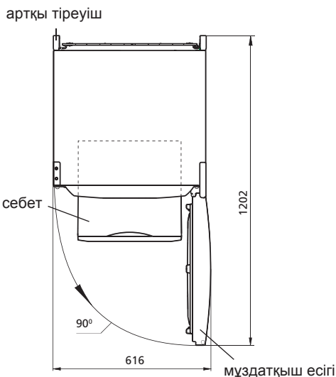
Сурет 2 – Мұздатқыш (түр үстіңгі жағынан)
